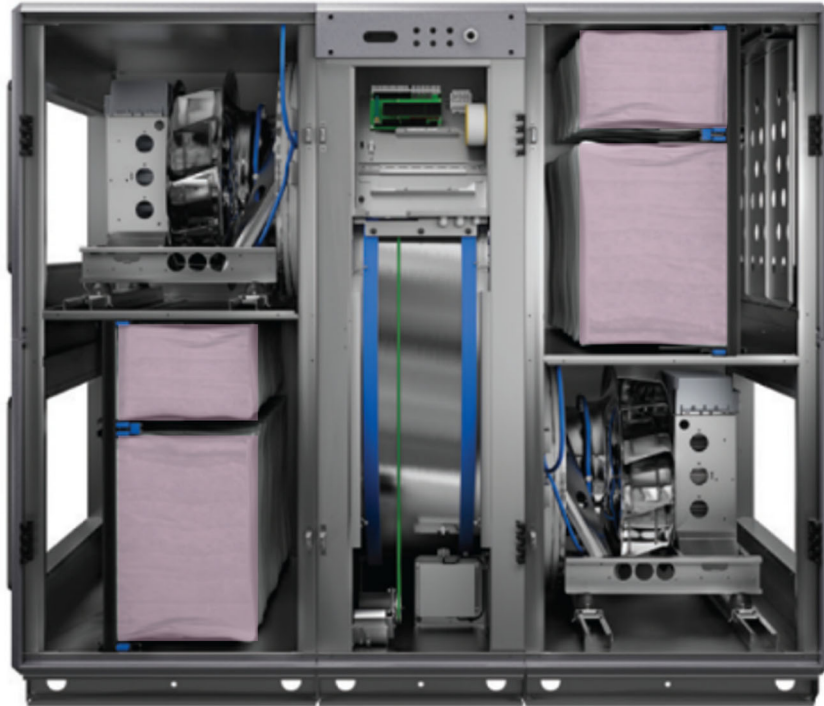
Figur 1, Typisk ventilasjonsaggregat med posefiltre før og etter varmegjenvinneren.
